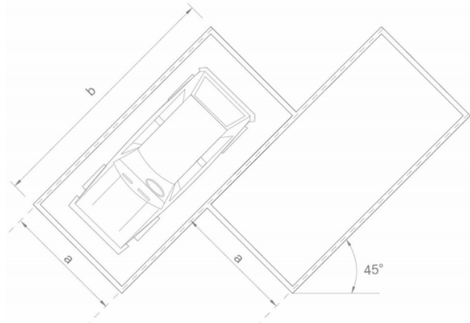
Figura 7. Plaza de estacionamiento 45°. Tomado de “CONADIS”. Recuperado de: https://drive.google.com/file/d/0Bxl4LLo2QyyJUHZOYXM1c0s2dzA/view?usp=drive_web
