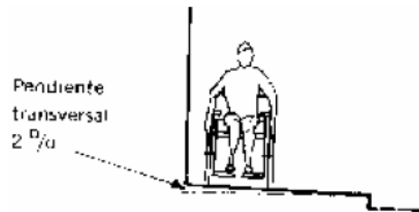
Figura 5. Pendientes transversal 2%. Tomado de “CONADIS”. Recuperado de: https://drive.google.com/file/d/0Bxl4LLo2QyyJcjUwRy05UzluRHc/view
