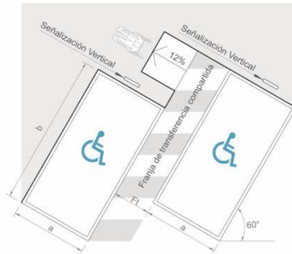
Figura 9. Plaza de estacionamiento para personas con discapacidad. Tomado de “CONADIS” Recuperado de: https://drive.google.com/file/d/0Bxl4LLo2QyyJUHZOYXM1c0s2dzA/view?usp=drive_web
