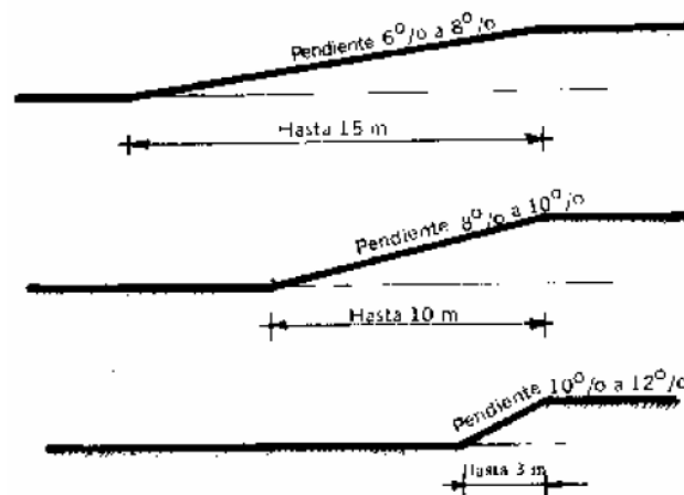
Figura 4. Pendientes longitudinales. Tomado de “CONADIS”. Recuperado de: https://drive.google.com/file/d/0Bxl4LLo2QyyJcjUwRy05UzluRHc/view
