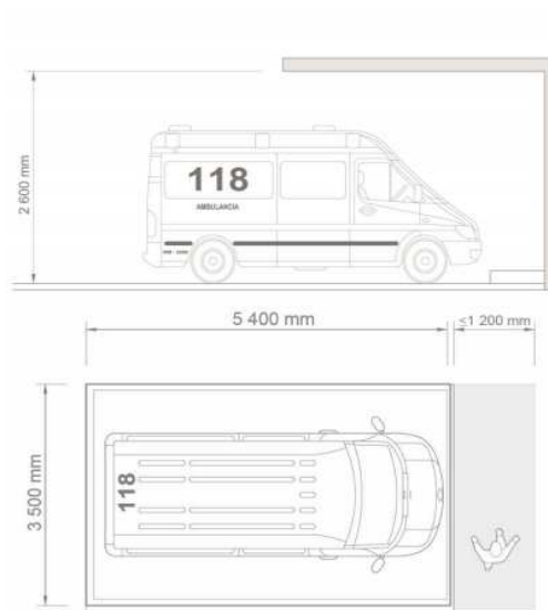
Figura 8. Estacionamiento para vehículos de emergencia. Tomado de “CONADIS”. Recuperado de: https://drive.google.com/file/d/0Bxl4LLo2QyyJUHZOYXM1c0s2dzA/view?usp=drive_web
