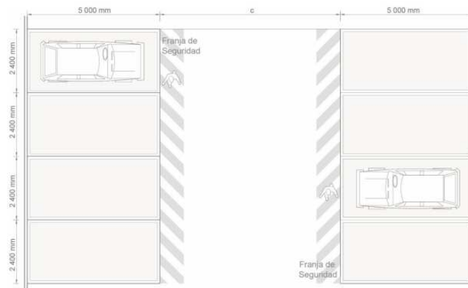
Figura 6. Franja de seguridad peatonal de uso preferencial. Tomado de “CONADIS”. Recuperado de: https://drive.google.com/file/d/0Bxl4LLo2QyyJUHZOYXM1c0s2dzA/view
